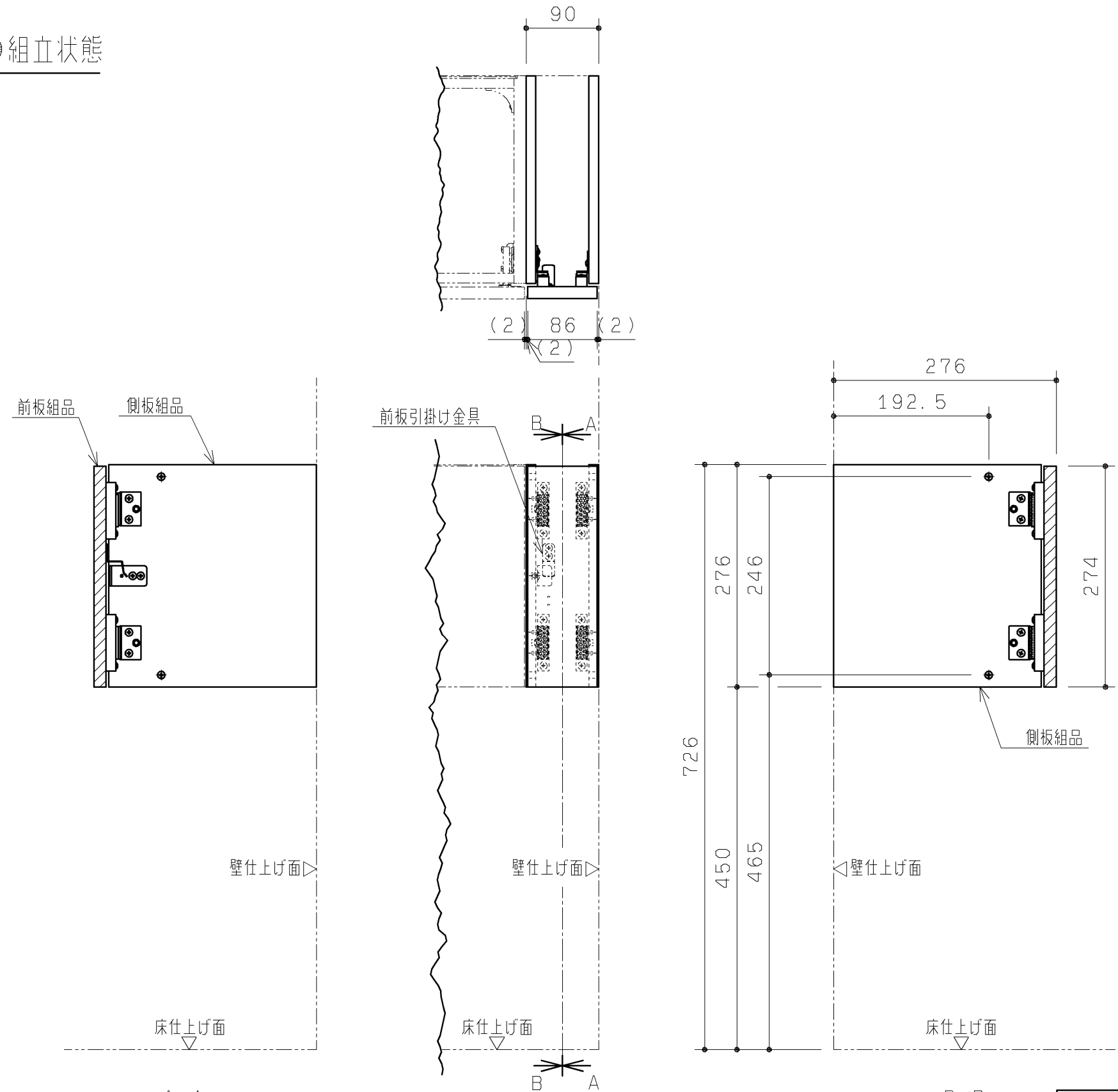
A-A キャビネット側
